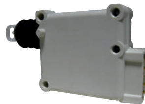
VALOR 0870 : MITSUBISHI L-300 SOL ÖN KAPI KİLİT MOTORU 1996-> 5 PİN OEM NO : 67301L / MB421491 / 528005570
