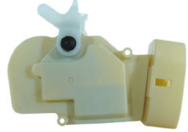
VALOR 0752 : ISUZU D-MAX SAG ÖN KAPI KİLİT MOTORU 2000->2005 OEM NO : 8973499930 / 6911030110 / 6911052010
