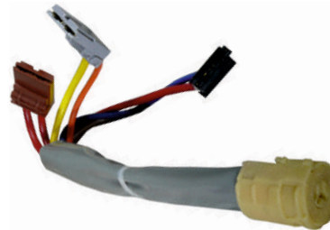
KA 1170 PEUGEOT 106 I / 106 II 1991-2001 PEUGEOT PARTNER 1992-1996 CITROEN SAXO 1998-> SERVIS NO : 416292 / 602795 / 252121
