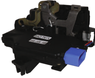
VALOR 0130 : JETTA/OCTAVIA / FABIA / TOLEDO / LEON SOL ÖN KAPI KİLİT MOTORU OEM NO : 3D1837015
