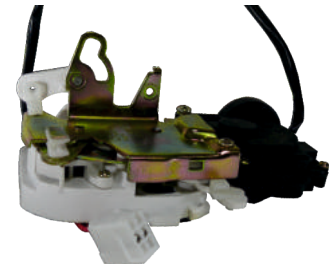
VALOR 0407 : MAZDA 323 SAG ÖN KAPI KİLİDİ KOMPLE MOTORLU 2 PİN OEM NO : BJ3D58310
