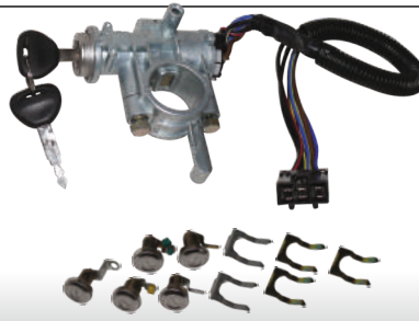
MI 690 MITSUBISHI L300 MİNİBUS / L300 PANELVAN 1988->1999 L300 KOMPLE KONTAK+ KAPI SIFRE TAKIMI OEM NO : MB364965 / MB541589
