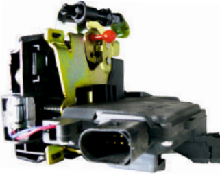
VALOR 0008 : AUDI A-3/AUDI A-4 SAG ARKA KAPI KİLİT MOTORU 7 PİN OEM NO : 8D0839016A / 8E0839016D
