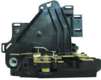
VALOR 0030 : SEAT CORDOBA / IBIZA IV / VW POLO SAĞ ARKA MERKEZİ KİLİT MOTORU 2002-2009 OEM NO : 3B1837016BR
