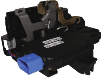
VALOR 0135 : JETTA / OCTAVIA / FABIA / TOLEDO / LEON SAĞ ÖN KAPI KİLİT MOTORU OEM NO : 3D1837016
