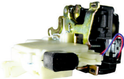
VALOR 0150 : VOLKSWAGEN JETTA / GOLF SOL ÖN KAPI KİLİT MOTORU 8 PİN OEM NO : 3B1837015AS / 3B1837015AK / 3B1837015J
