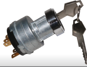
KA 0020 DODGE / DESOTO / FARGO S100 / S200 / AS250 / AS400 / AS600 / AS700 / AS800 / AS900 1969->2000 MARS LI KONTAK OEM NO : 2097628 / 2497158 / 2864258 / WELLS LS472
