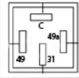
VF 295 24VOLT 4PIN OTOYOL IVECO / VOLVO FLASOR OEM NO : 41730537 / 0288326 / 11087239 / 53401102
