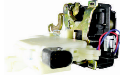
VALOR 0154 : VOLKSWAGEN JETTA / GOLF SOL ARKA KAPI KİLİT MOTORU 6 PİN OEM NO : 3B4839015AM
