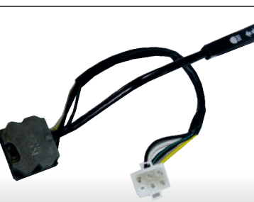
SS 884 VOLVO TD100 SELLEKTÖR / SİNYAL KOLU 5PİN OEM NO : 201095 / 1501805
