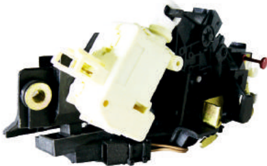
VALOR 0066 : AUDI A-6 BAGAJ KİLİDİ MOTORLU KOMPLE 2000-> 4 PİN OEM NO : 4B0827565J
