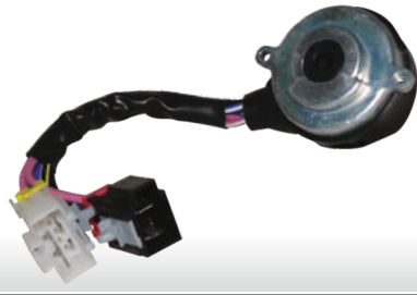
MI 630 MITSUBISHI CANTER FE511 / CANTER FE659 / CANTER FE659E TURBO 1998->2005 YENİ MODEL KONTAK TERMINALI SERVIS NO : MC8985741
