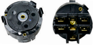
KA 1120 FIAT PALIO 1996- > / FIAT SIENA 1998-> PEUGEOT BOXER 1994-> CITROEN JUMPER 1995-> OEM NO : 72697802 SERVIS NO : Q215A7
