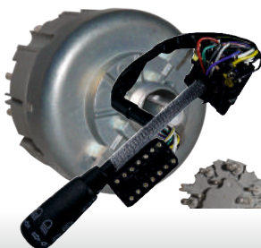
ME 40 MERCEDES W124 KASA 1985->1996 FAR ANAHTARI OEM NO : 0005456204
