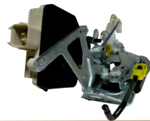
VALOR 0834 : HYUNDAI ELENTRA SOL ARKA KAPI KİLİDİ KOMPLE MOTORLU 2001-> 5 PİN OEM NO : 814102D001
