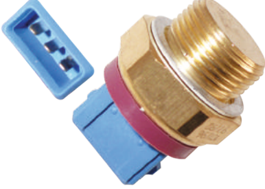
VFM 0030 PEUGEOT PARTNER 1.9D / 306 / CITROEN BERLINGO / XSARA 1.9D 3 FİŞLİ 1993->2001 FAN MUSURU 87°C / 92°C -> 92°C / 97°C OEM NO : 126425 / 126438 / 126445 / 96064750 / 819747
